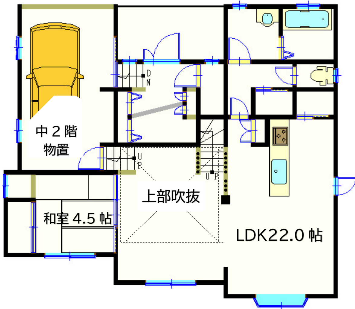
1 階平面図 床面積:26.75 坪 (ガレージ 5.25 坪含む)
